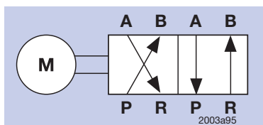
Umsteuerung (4/2-Wegeventil)
