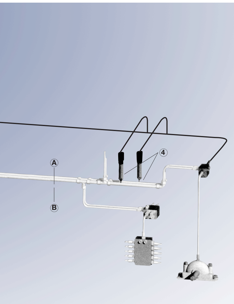
Schemazeichnung Zweileitungsanlage (konventionelle Anlage)
