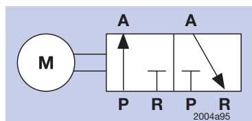
3/2-Wegeventil Anschluss B geschlossen
